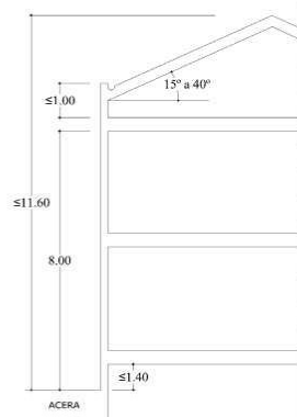
CON APROVECHAMIENTO BAJO CUBIERTA Y SEMISÓTANO
