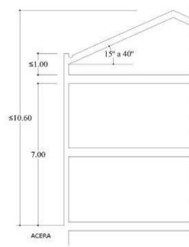
CON APROVECHAMIENTO BAJO CUBIERTA Y SIN SEMISÓTANO
