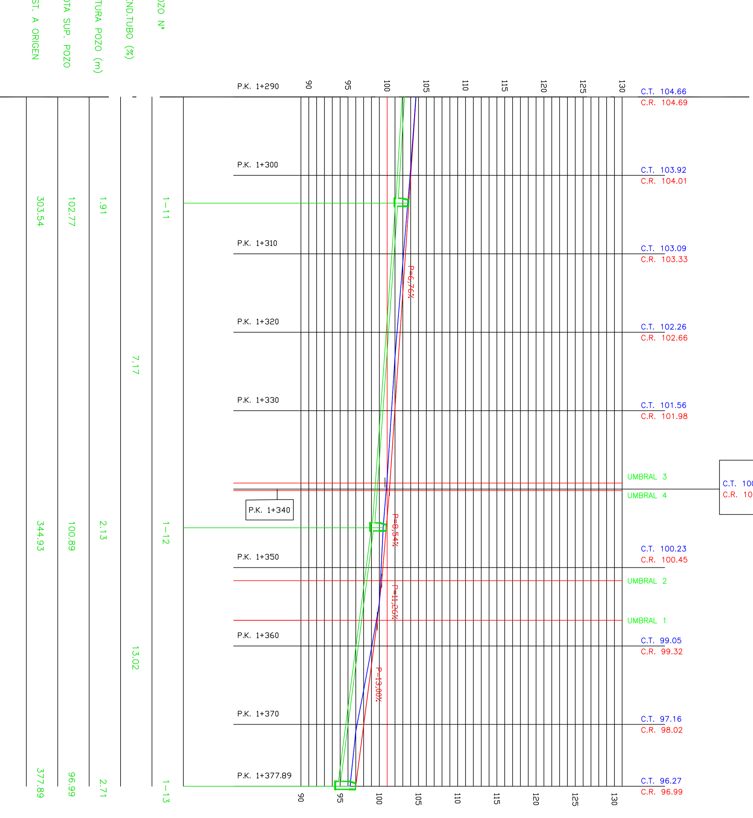
SECCION LONGITUDINAL a-a' Escala: 1/200
